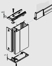
Montaż we wnęce.
