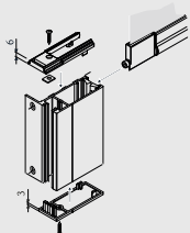
Montaż we wnęce.
