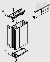
Befestigung in der Nische
