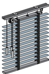
Breite: max. 270 cm Höhe: max. 300 cm Bedienungsoptionen: Schnur-Schnur, Schnur-Stab Befestigung: Wand, Decke und Fensternische.
