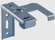
Universal-Träger (TWIST) Wand- oder Deckenbefestigung
